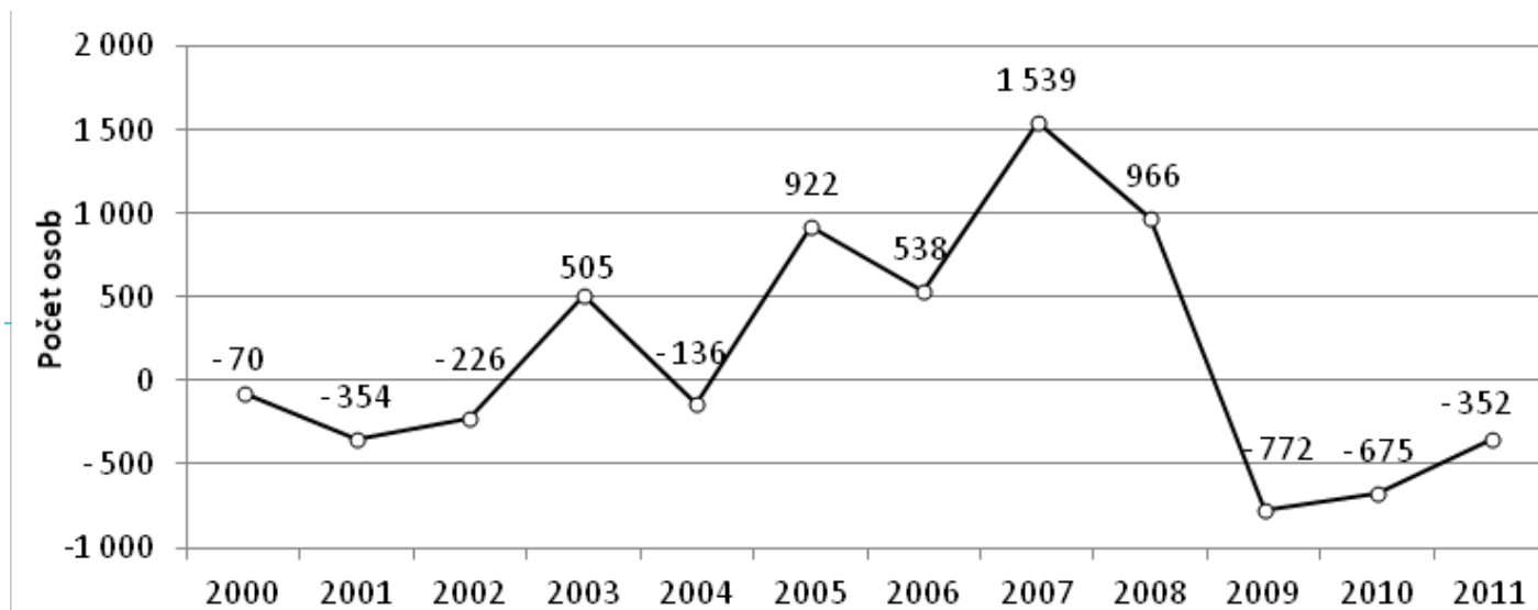
Obr. 1: Vývoj migračního salda Kraje Vysočina v letech 2000–2011
