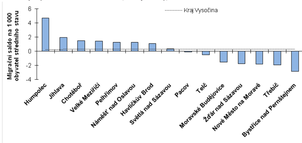
Obr. 2: Hrubá míra migračního salda ve správních obvodech ORP Kraje Vysočina v letech 2000–2011 (roční průměry)
